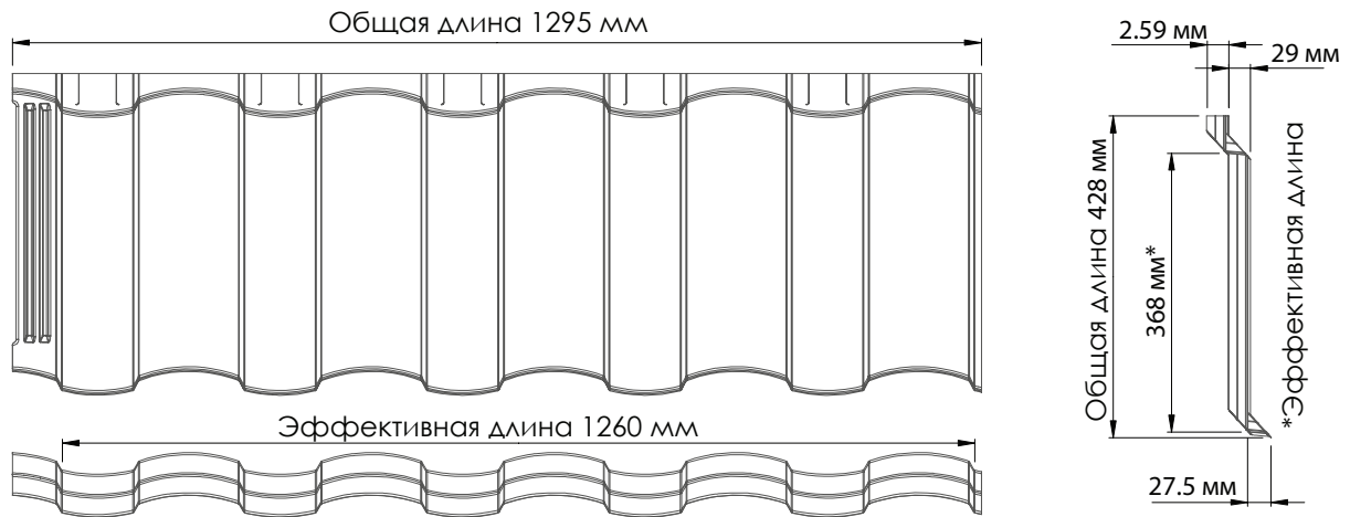
Рис. 8.1 Размеры профиля
