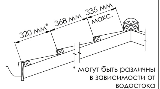
Рис. 5.5 Расположение реек обрешетки
