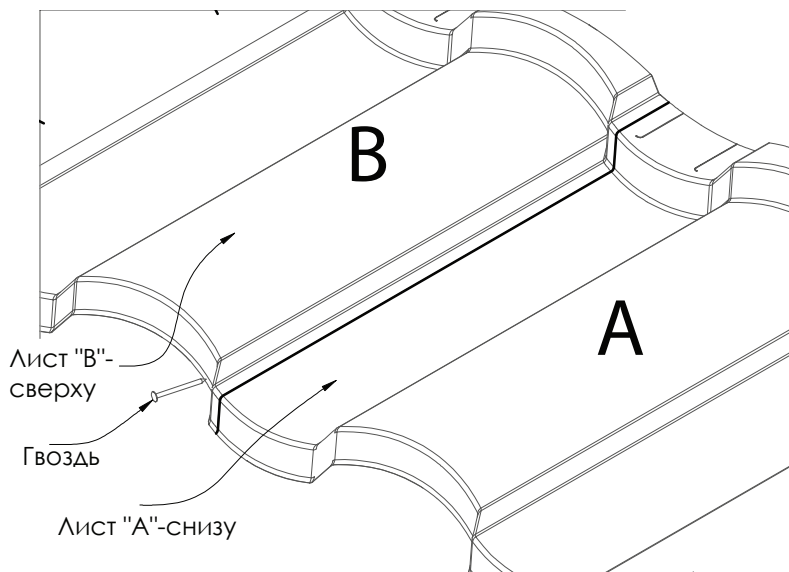
Рис. 5.3 Перекрытие листов
