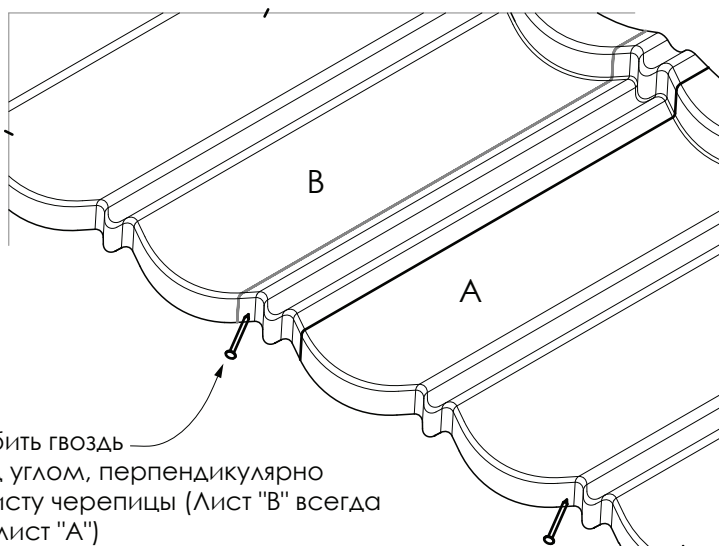
Рис. 1.3 Перекрытие листов
