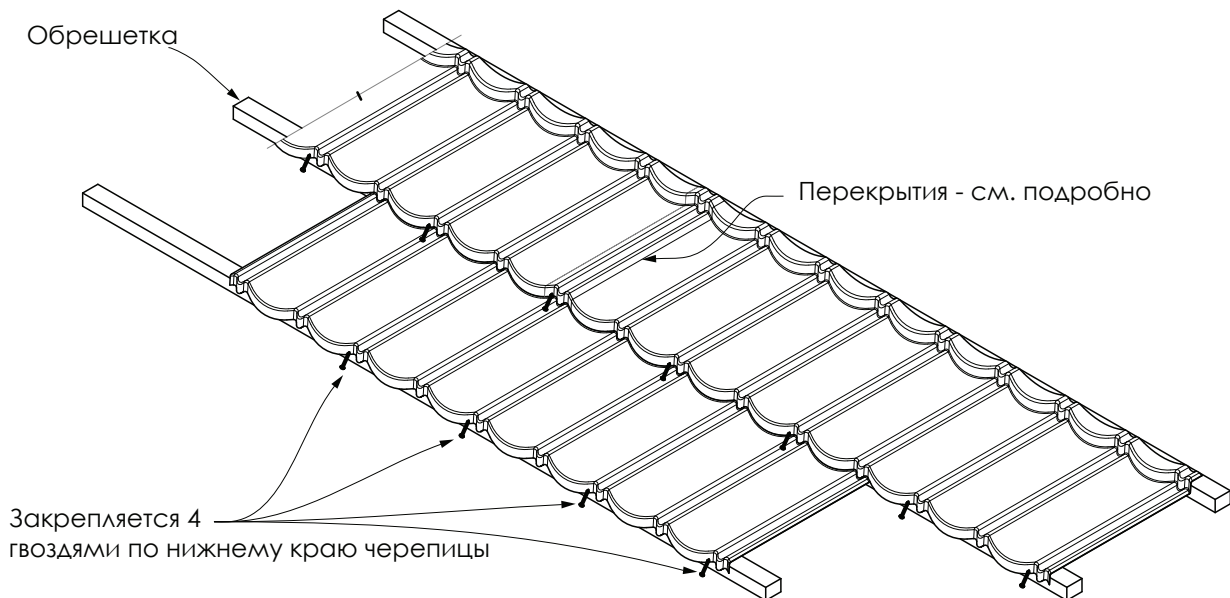
Рис. 1.2 Крепление гвоздей
