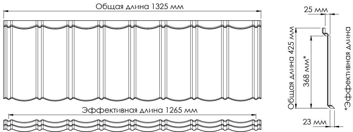
Рис. 1.1 Размеры профиля
