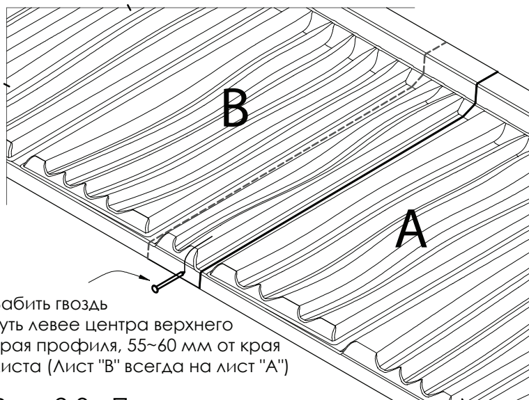
Рис. 2.3 Перекрытие листов
