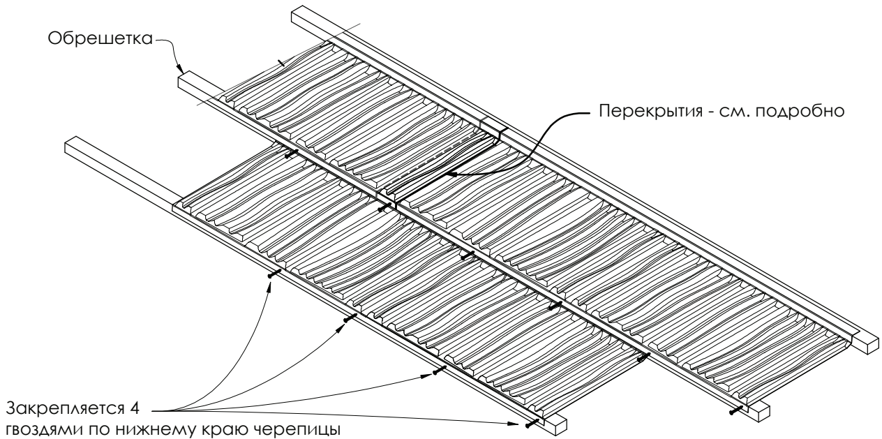
Рис. 2.2 Крепление гвоздей
