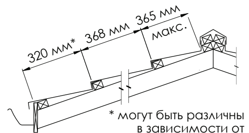
Рис. 2.5 Расположение реек обрешетки
