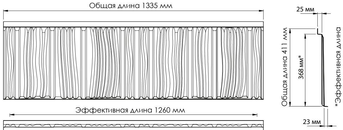
Рис. 2.1 Размеры профиля
