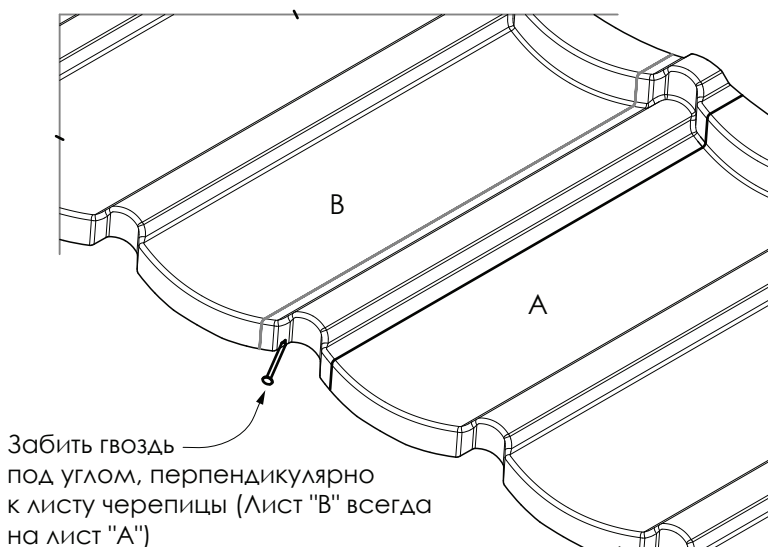
Рис. 6.3 Перекрытие листов
