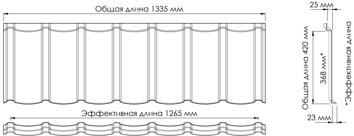
Рис. 6.1 Размеры профиля
