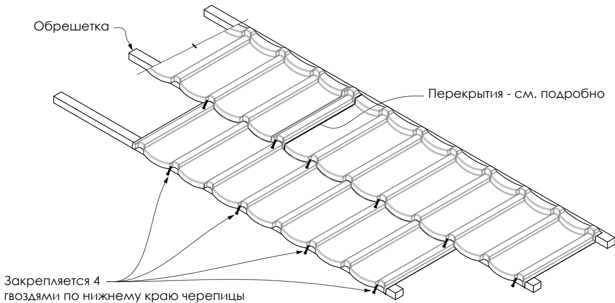
Рис. 6.2 Крепление гвоздей
